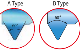
나사산 확대
