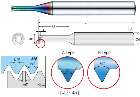
나사산 확대
